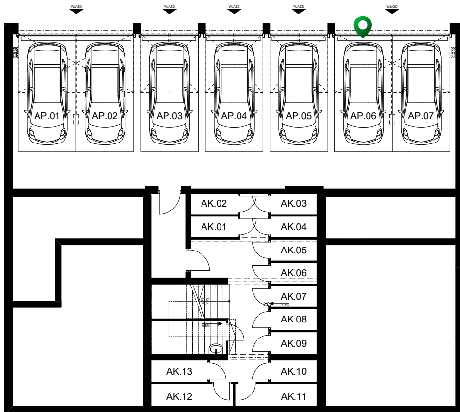
Rzut garażu budynku A
